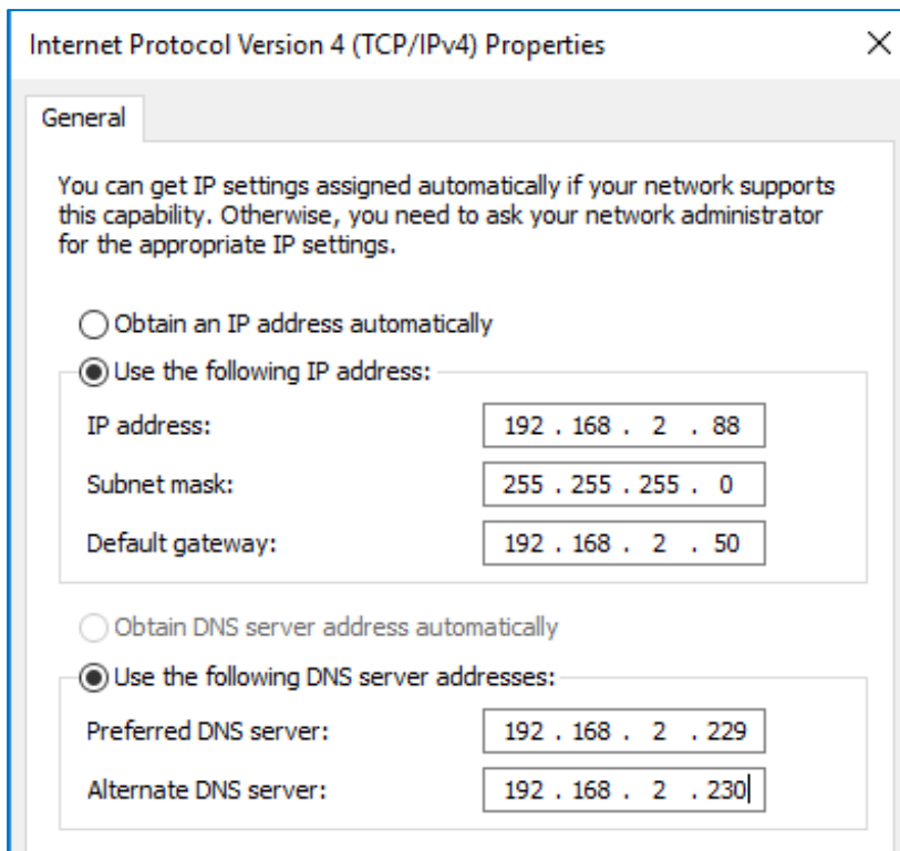
Figura 9. Konfigurimi i IP së hostit Windows, PSM
